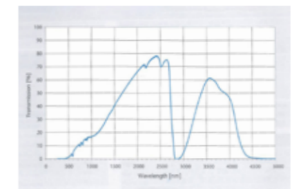
Strahlungsdurchlässigkeit weißes Glas
