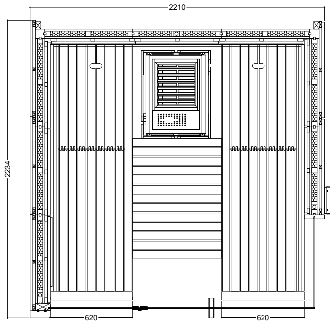
Aufbau links
