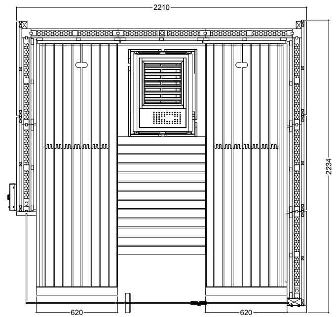
Aufbau rechts
